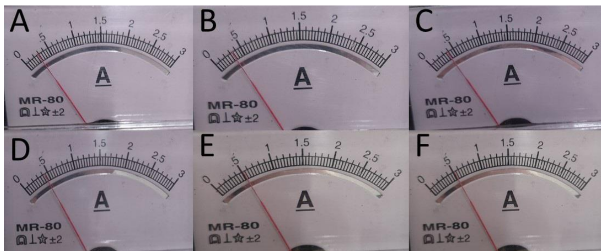
4 pav. Ampermetro rodmenys keičiant šliaužiklinio reostato slankiklio padėtį.
